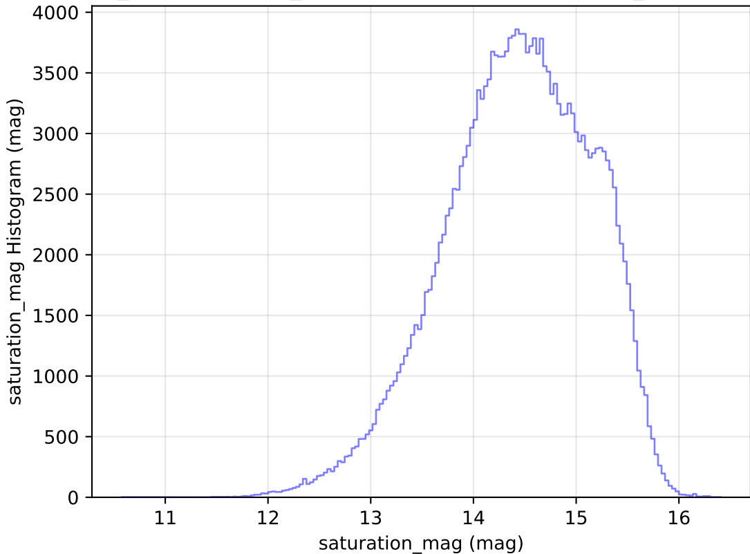
weather_cloudso14v3.4_10yrs WFD g band: saturation_mag Histogram
