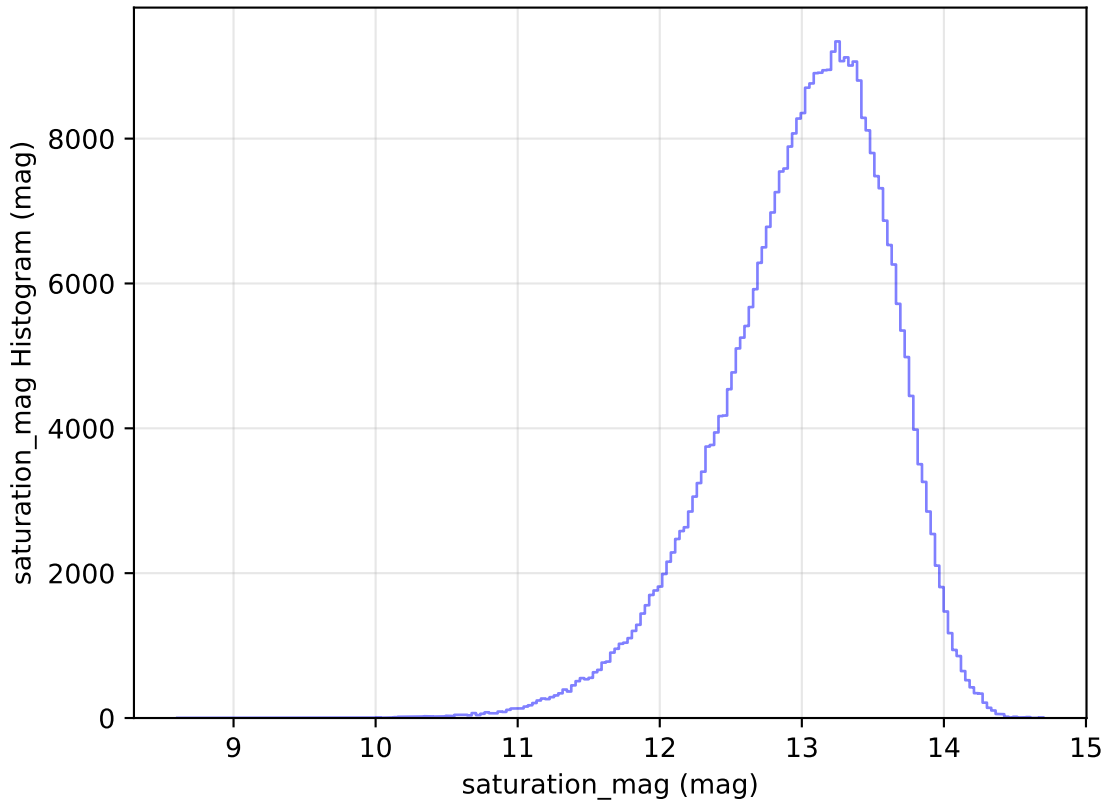
weather_cloudso14v3.4_10yrs All sky y band: saturation_mag Histogram
