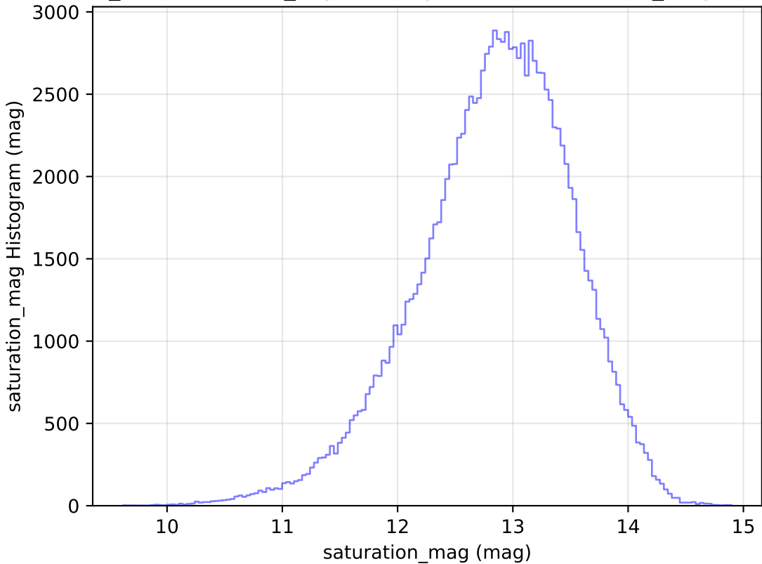
weather_cloudso14v3.4_10yrs All sky u band: saturation_mag Histogram
