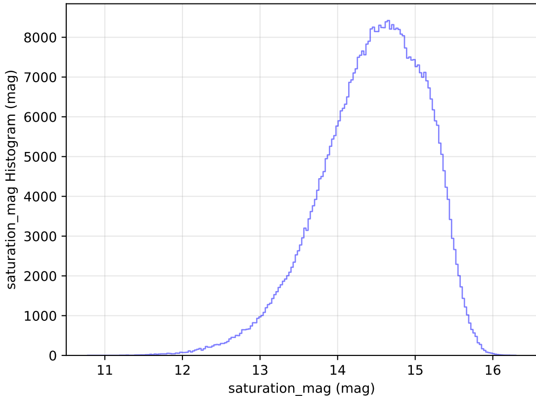
weather_cloudso14v3.4_10yrs All sky r band: saturation_mag Histogram
