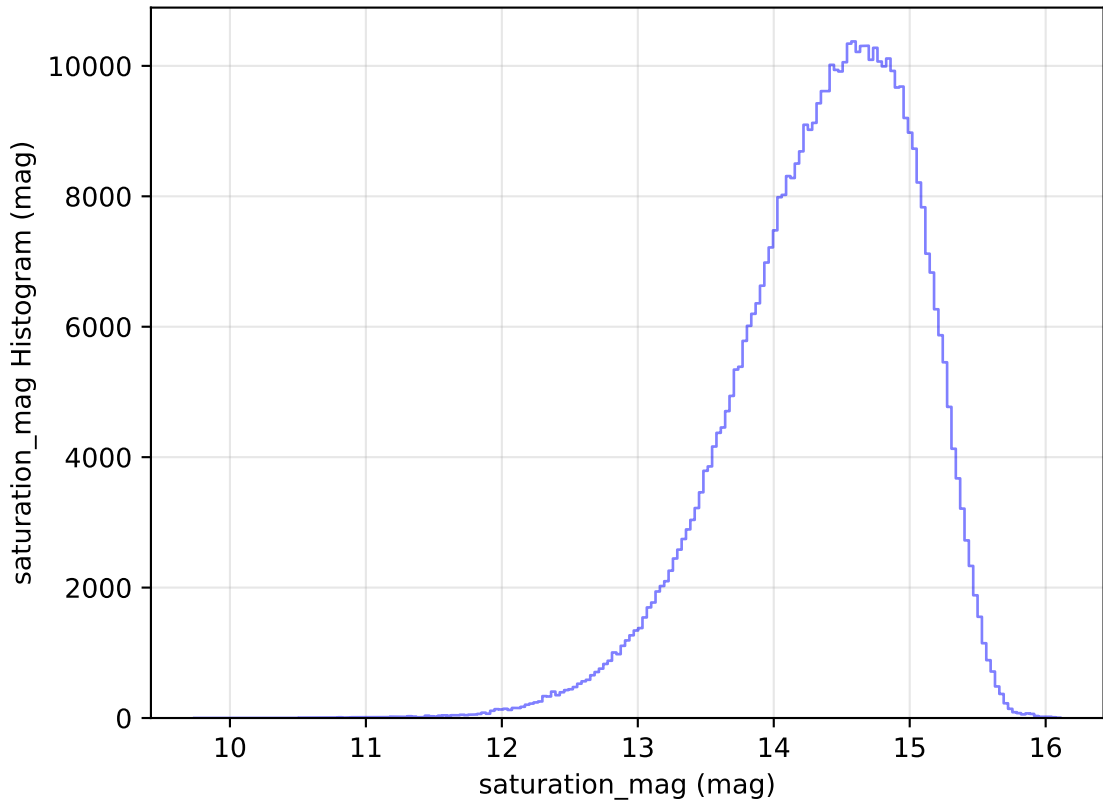
weather_cloudso14v3.4_10yrs All sky i band: saturation_mag Histogram
