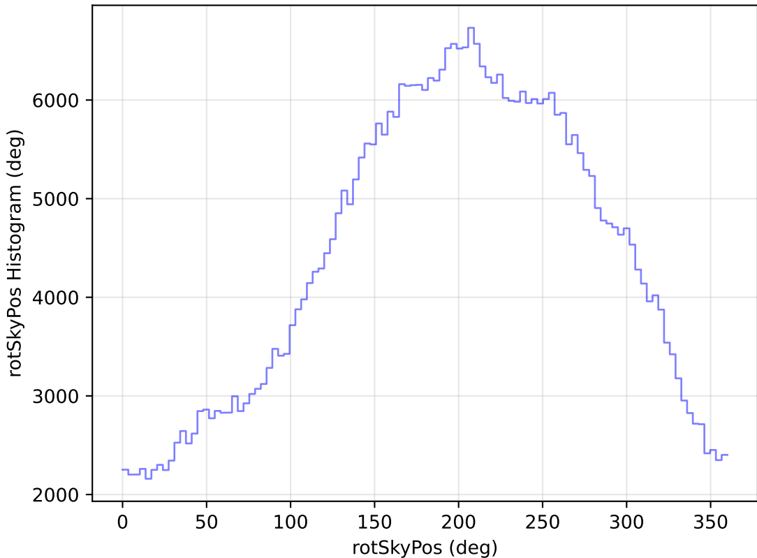
weather_cloudso14v3.4_10yrs WFD z band: rotSkyPos Histogram
