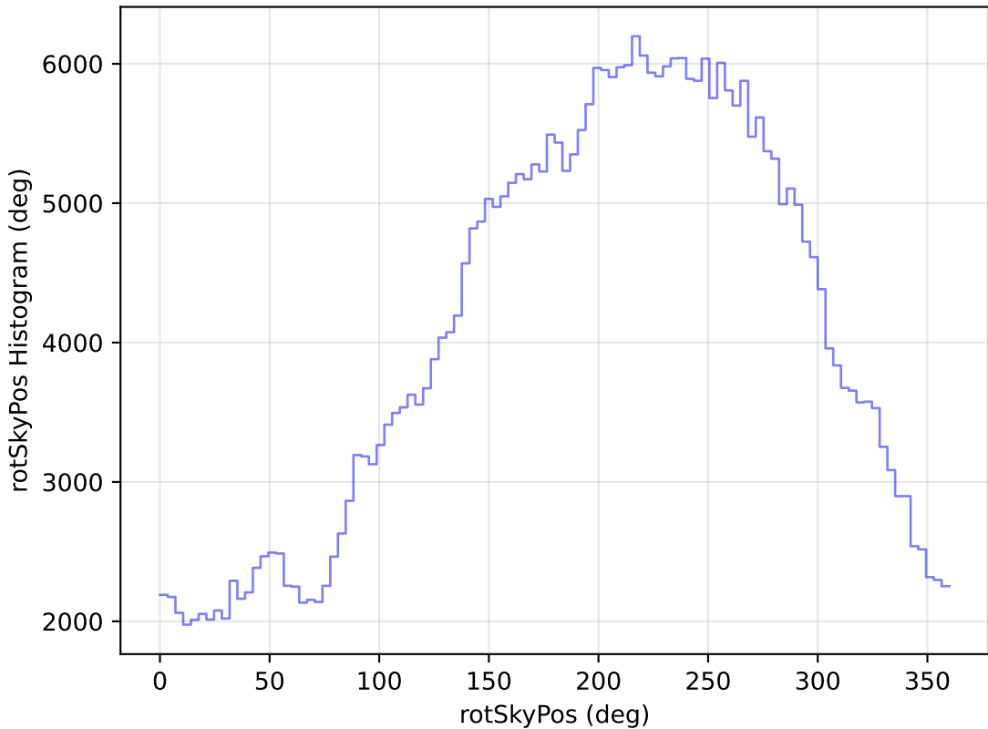
weather_cloudso14v3.4_10yrs WFD y band: rotSkyPos Histogram
