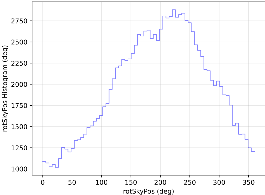
weather_cloudso14v3.4_10yrs WFD u band: rotSkyPos Histogram
