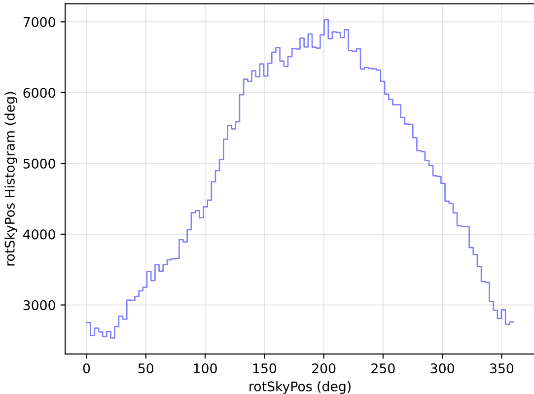
weather_cloudso14v3.4_10yrs WFD r band: rotSkyPos Histogram
