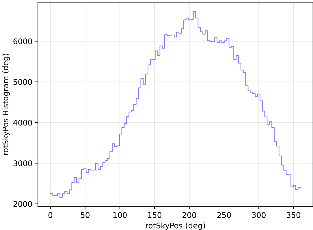
weather_cloudso14v3.4_10yrs All sky z band: rotSkyPos Histogram
