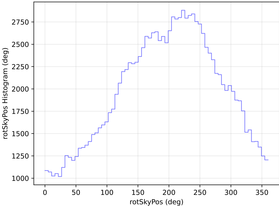
weather_cloudso14v3.4_10yrs All sky u band: rotSkyPos Histogram
