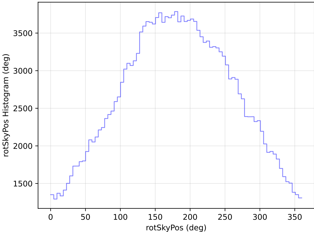
weather_cloudso14v3.4_10yrs All sky g band: rotSkyPos Histogram
