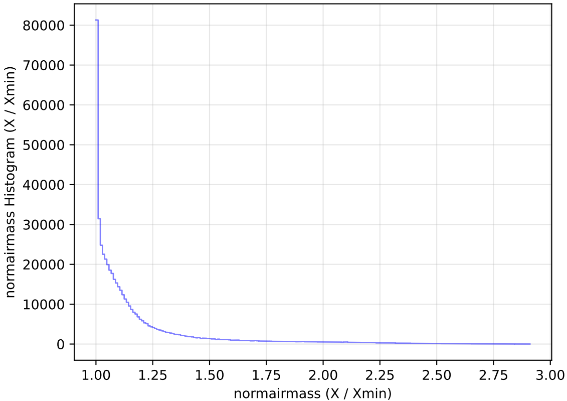
weather_cloudso14v3.4_10yrs All sky i band: normairmass Histogram
