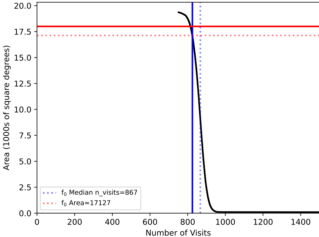
weather_cloudso14v3.4_10yrs WFD: fO
