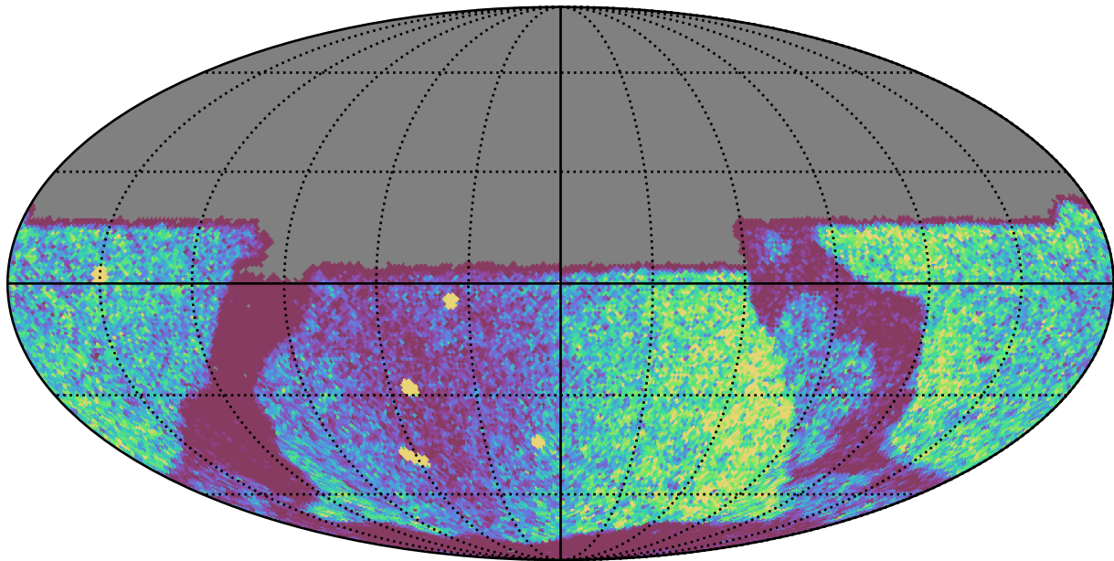
weather_cloudso14v3.4_10yrs Yr 1 y band: NVisits
