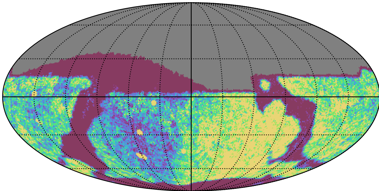
weather_cloudso14v3.4_10yrs Yr 1 i band: NVisits
