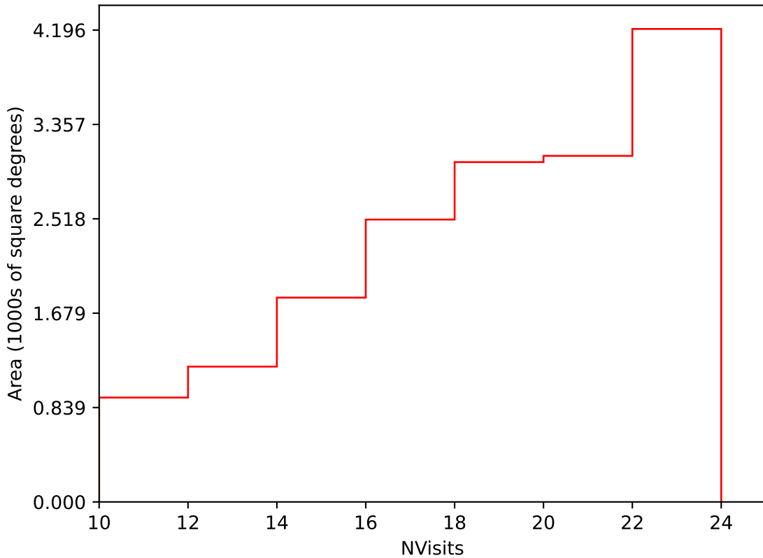
weather_cloudso14v3.4_10yrs Yr 1 i band: NVisits
