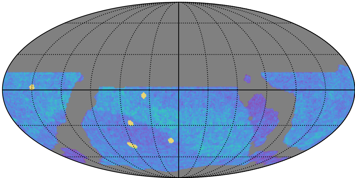
weather_cloudso14v3.4_10yrs WFD z band: NVisits
