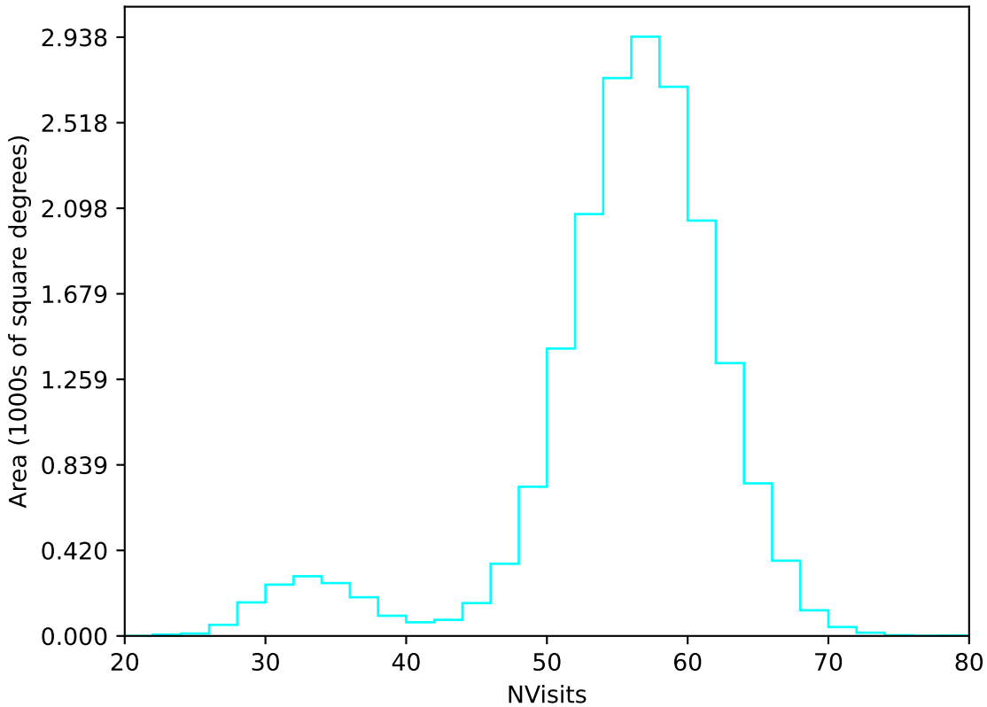
weather_cloudso14v3.4_10yrs WFD u band: NVisits
