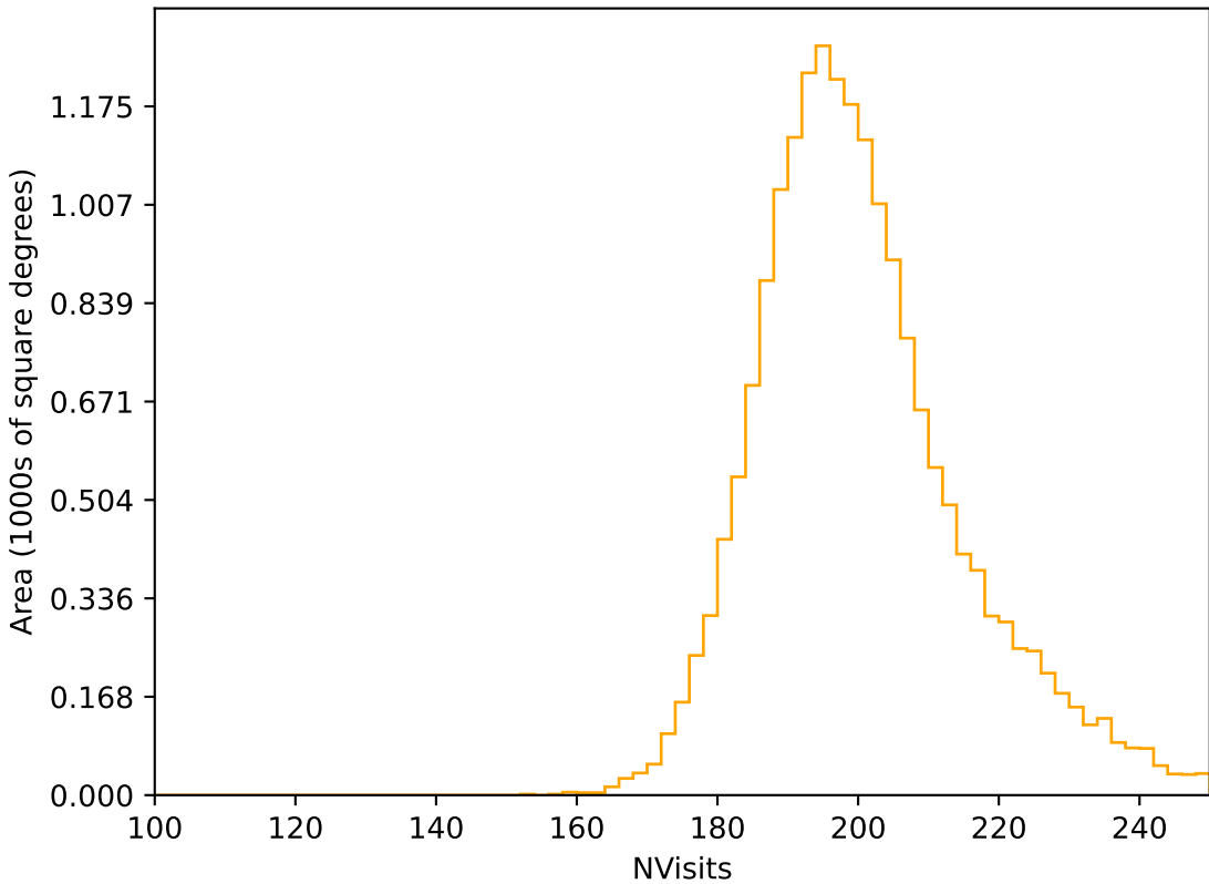
weather_cloudso14v3.4_10yrs WFD r band: NVisits
