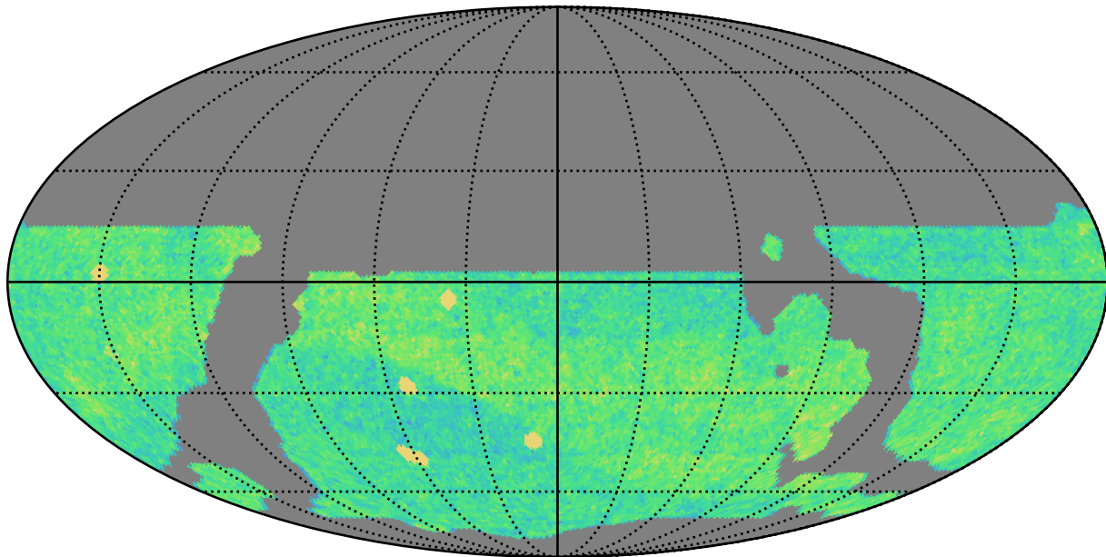
weather_cloudso14v3.4_10yrs WFD i band: NVisits
