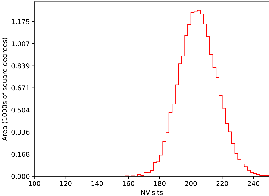
weather_cloudso14v3.4_10yrs WFD i band: NVisits
