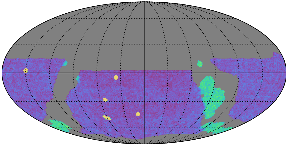
weather_cloudso14v3.4_10yrs WFD g band: NVisits
