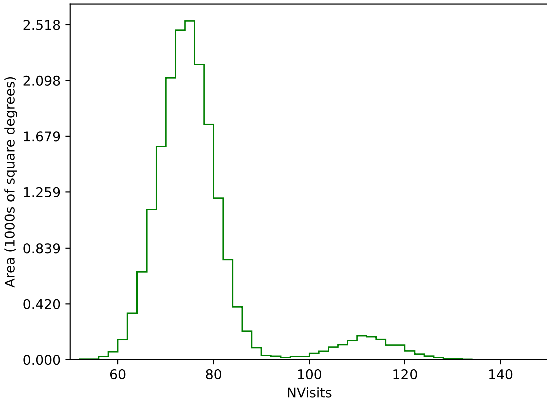
weather_cloudso14v3.4_10yrs WFD g band: NVisits
