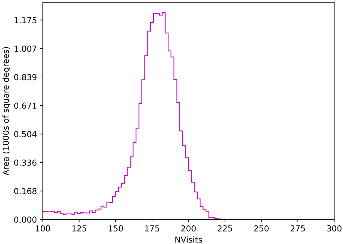
weather_cloudso14v3.4_10yrs All sky z band: NVisits
