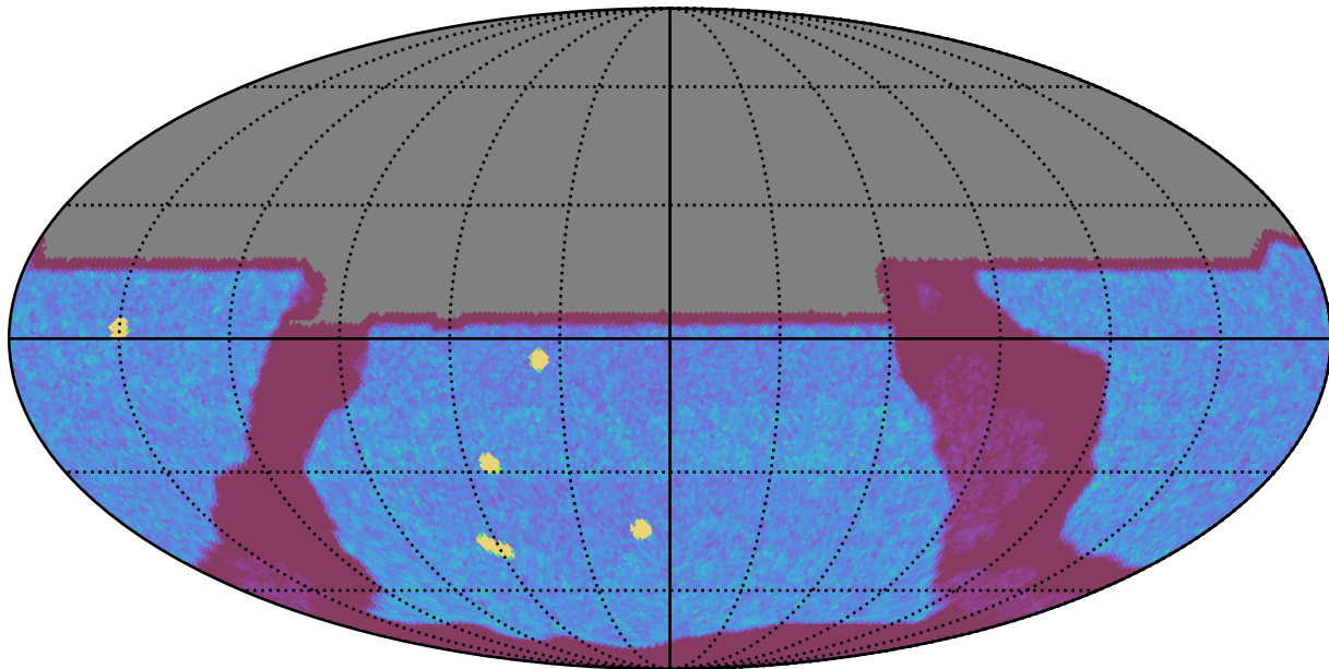
weather_cloudso14v3.4_10yrs All sky y band: NVisits
