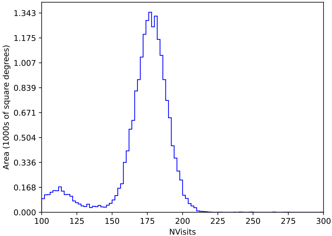
weather_cloudso14v3.4_10yrs All sky y band: NVisits
