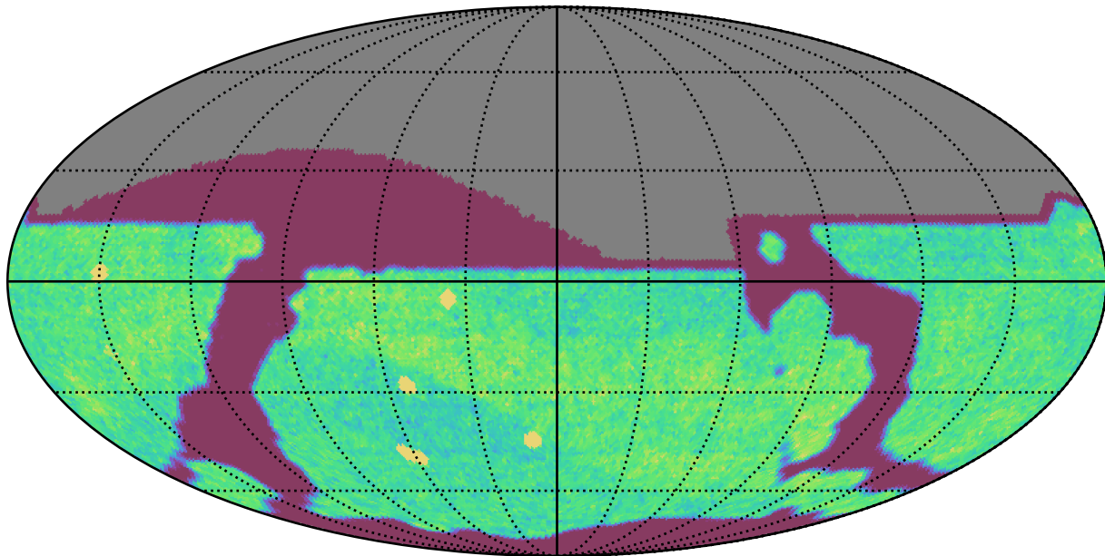
weather_cloudso14v3.4_10yrs All sky i band: NVisits
