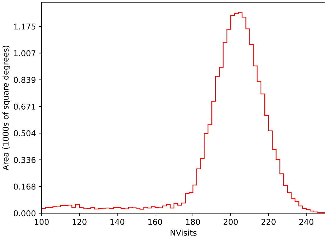
weather_cloudso14v3.4_10yrs All sky i band: NVisits
