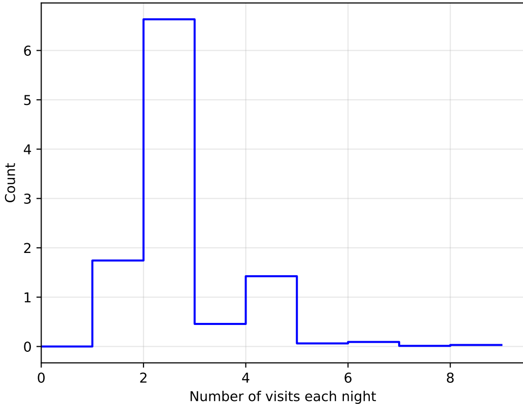
weather_cloudso14v3.4_10yrs All sky: NVisitsPerNight
