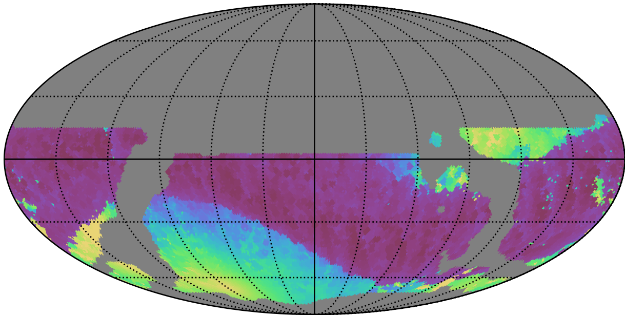
weather_cloudso14v3.4_10yrs WFD z band: Min solarElong
