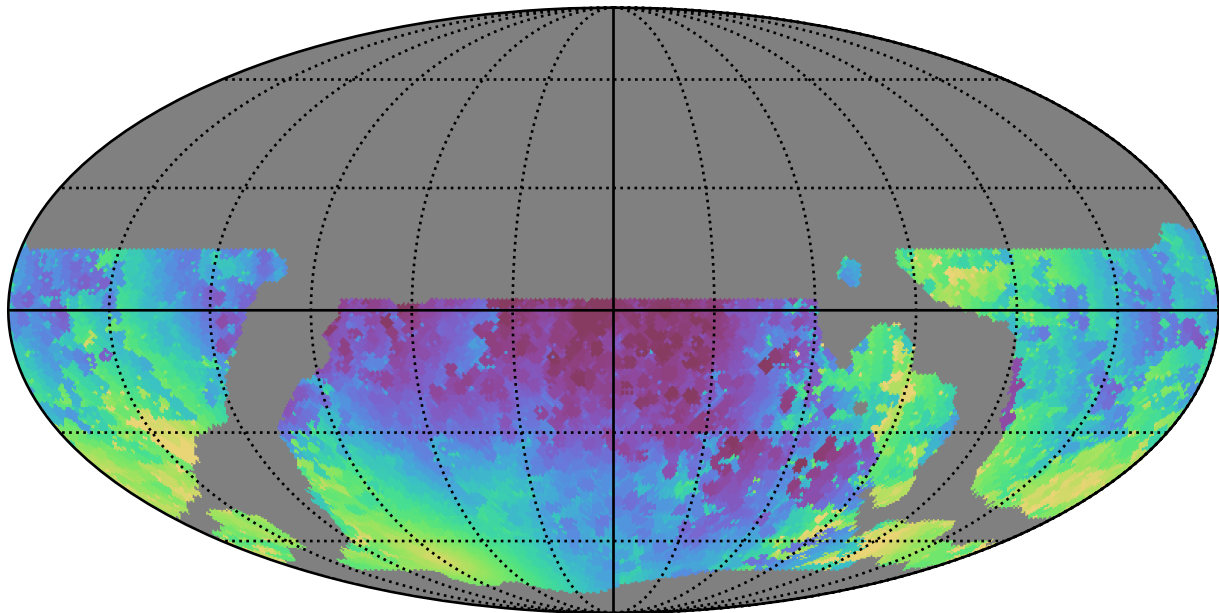
weather_cloudso14v3.4_10yrs WFD y band: Min solarElong
