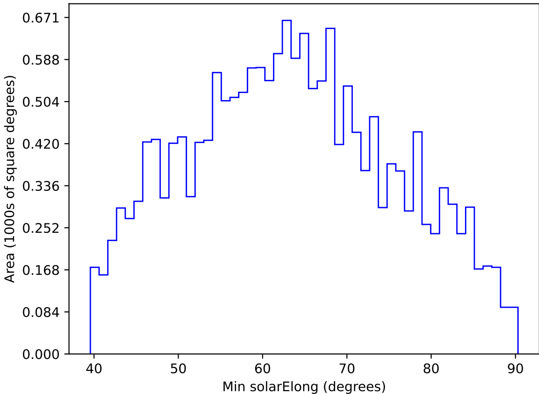
weather_cloudso14v3.4_10yrs WFD y band: Min solarElong
