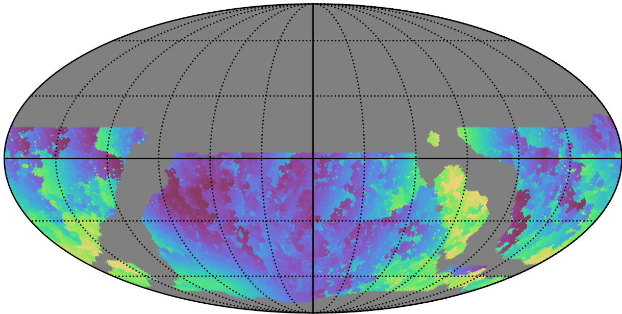
weather_cloudso14v3.4_10yrs WFD u band: Min solarElong
