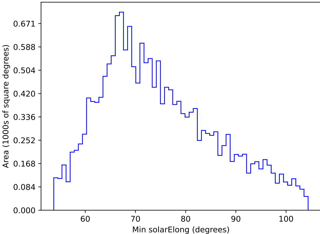
weather_cloudso14v3.4_10yrs WFD u band: Min solarElong
