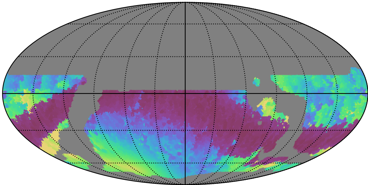
weather_cloudso14v3.4_10yrs WFD r band: Min solarElong
