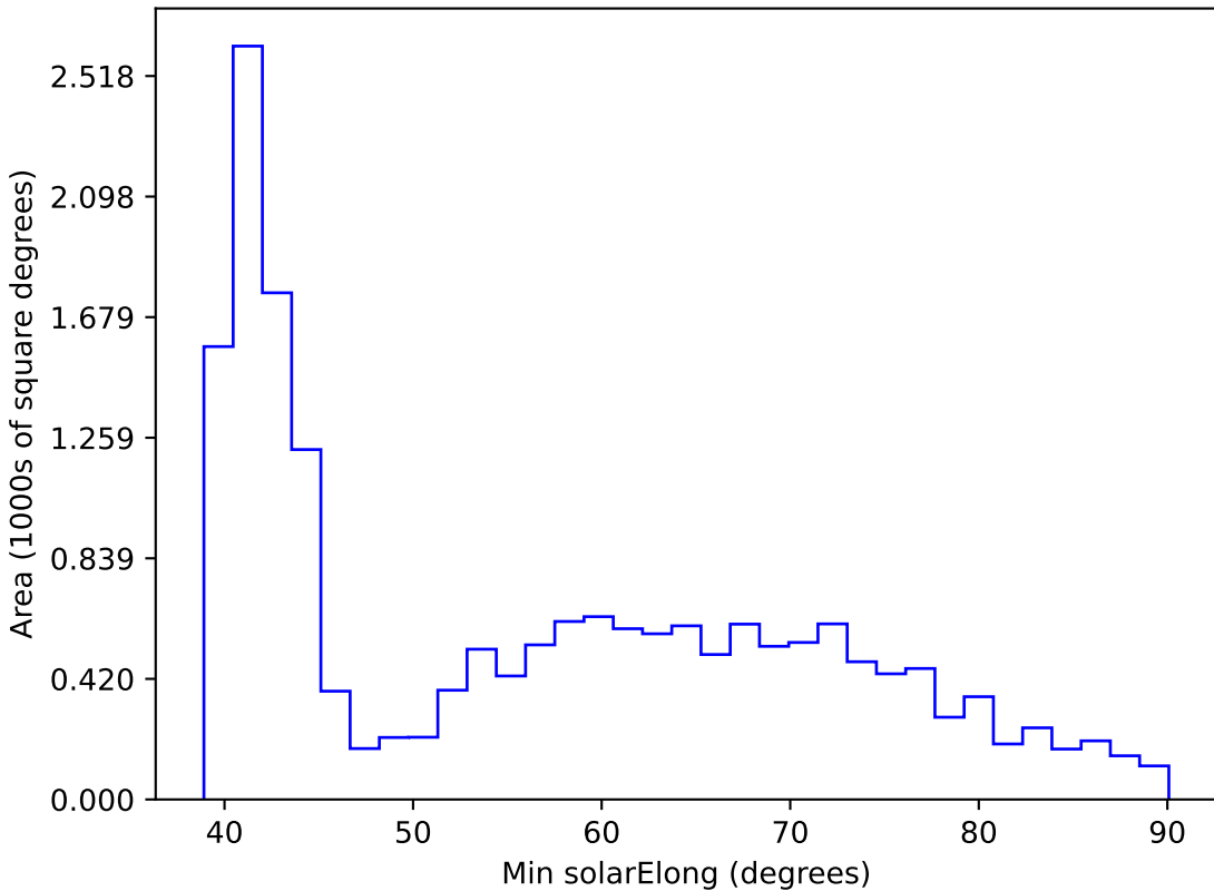
weather_cloudso14v3.4_10yrs WFD r band: Min solarElong
