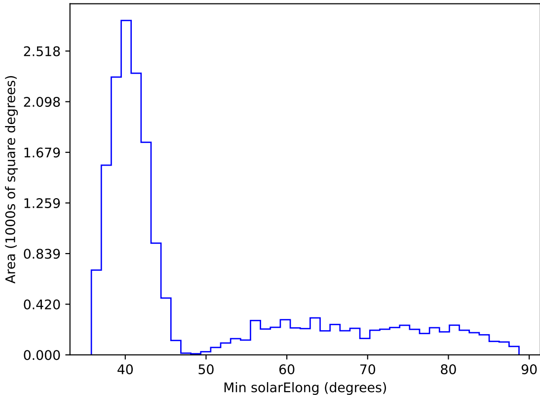
weather_cloudso14v3.4_10yrs WFD i band: Min solarElong
