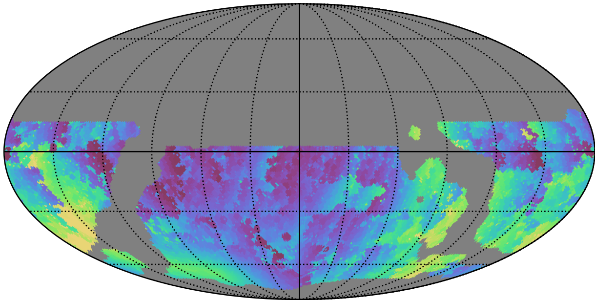
weather_cloudso14v3.4_10yrs WFD g band: Min solarElong
