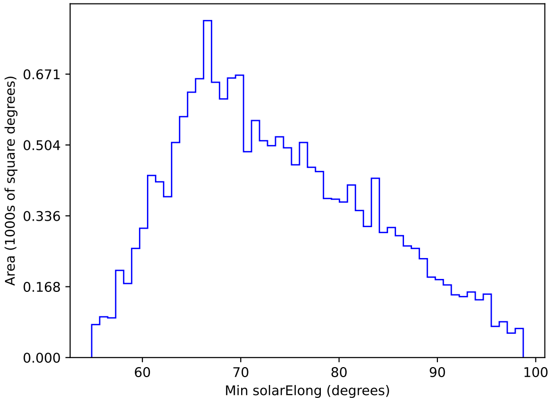
weather_cloudso14v3.4_10yrs WFD g band: Min solarElong
