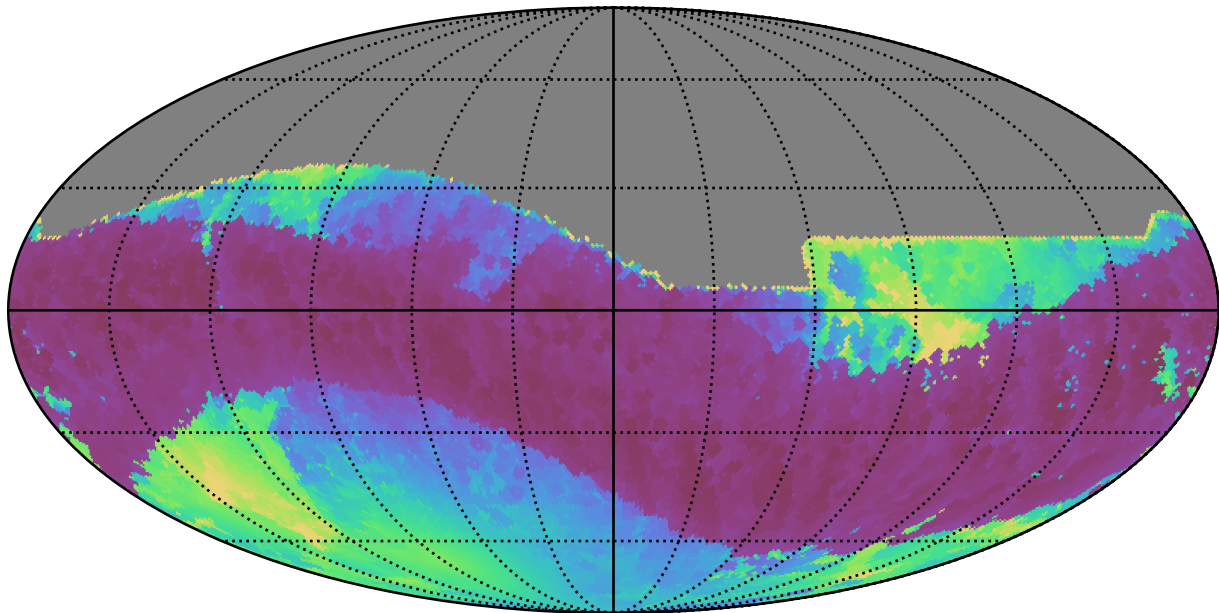
weather_cloudso14v3.4_10yrs All sky z band: Min solarElong
