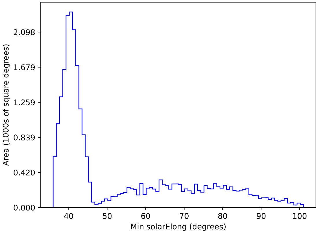
weather_cloudso14v3.4_10yrs All sky z band: Min solarElong
