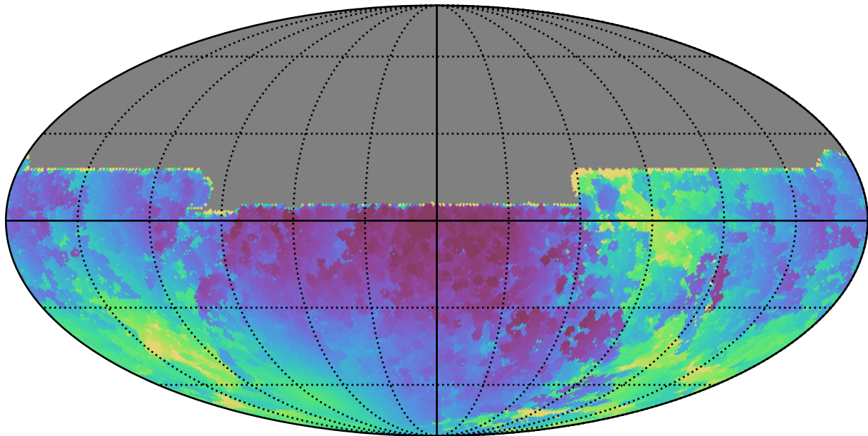
weather_cloudso14v3.4_10yrs All sky y band: Min solarElong
