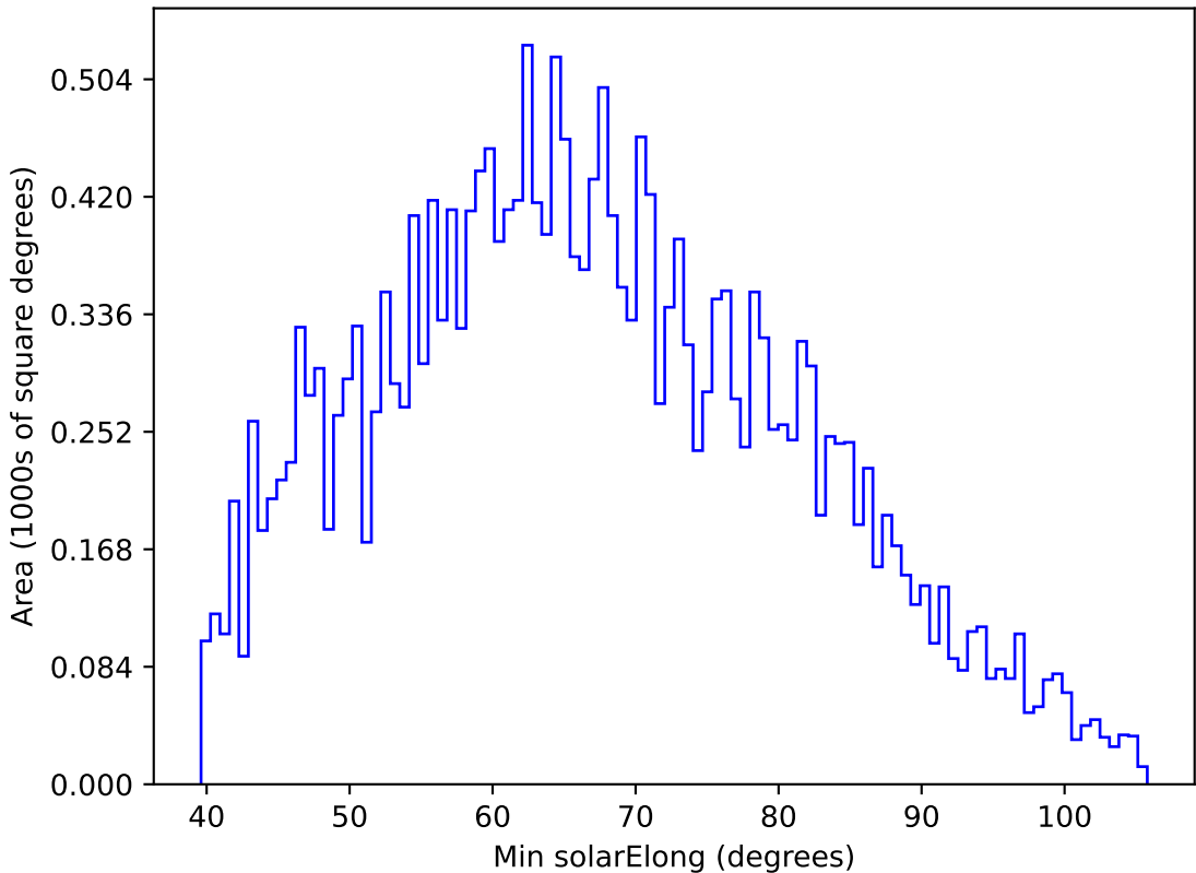
weather_cloudso14v3.4_10yrs All sky y band: Min solarElong
