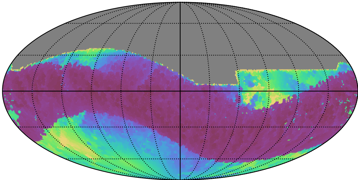
weather_cloudso14v3.4_10yrs All sky i band: Min solarElong
