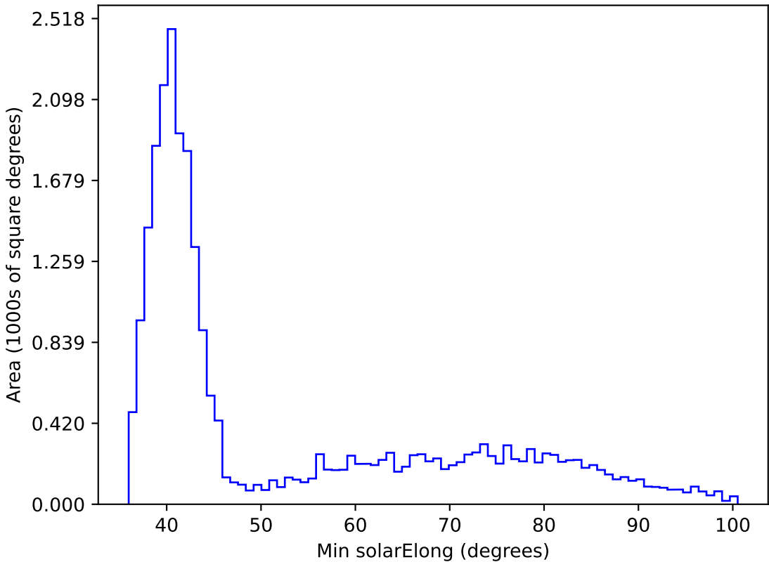
weather_cloudso14v3.4_10yrs All sky i band: Min solarElong
