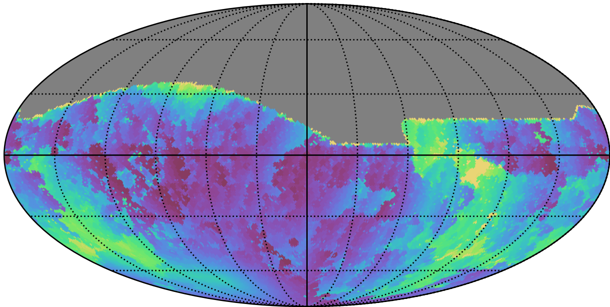
weather_cloudso14v3.4_10yrs All sky g band: Min solarElong
