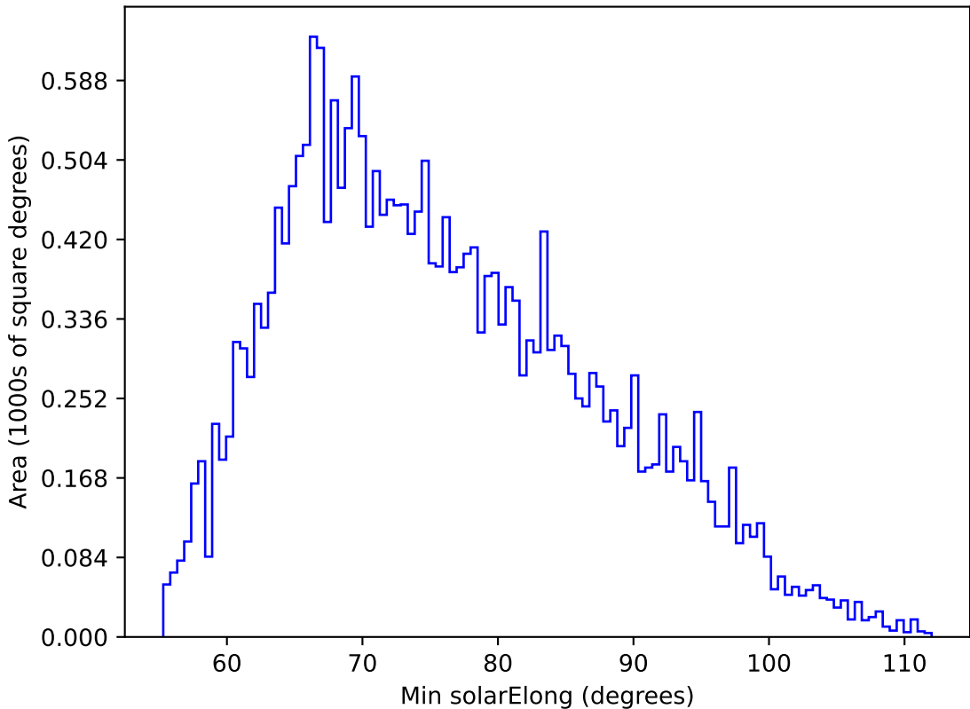
weather_cloudso14v3.4_10yrs All sky g band: Min solarElong
