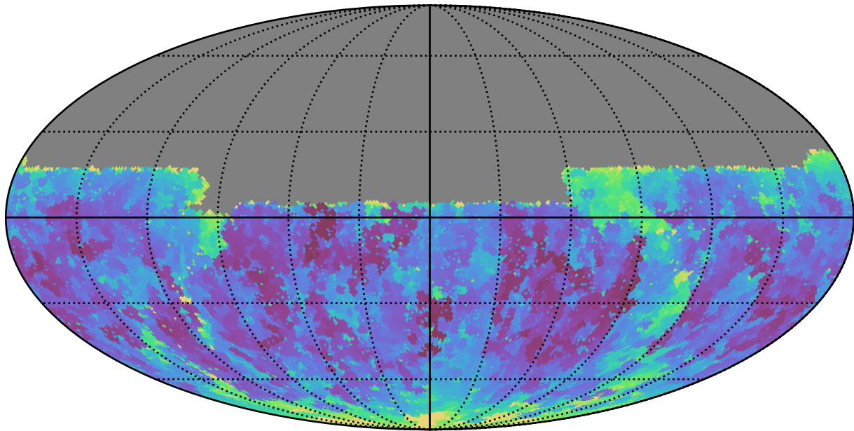
weather_cloudso14v3.4_10yrs Yr 1 y band: Min seeingEff
