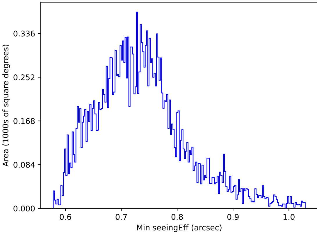
weather_cloudso14v3.4_10yrs Yr 1 y band: Min seeingEff
